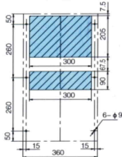
ZT-05开口图
